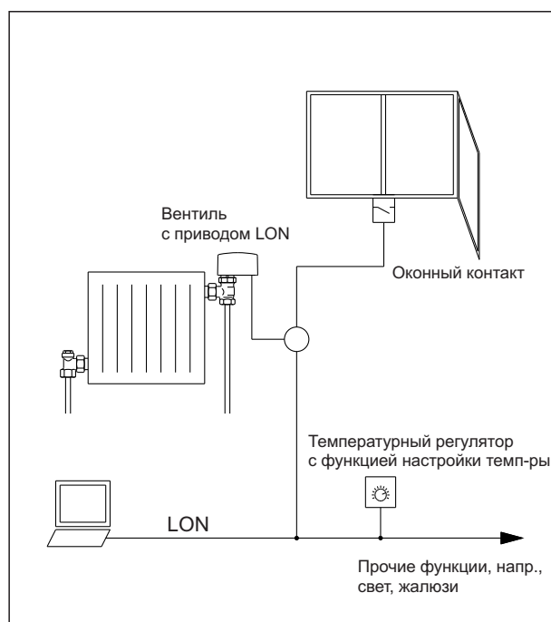
Пример установки
