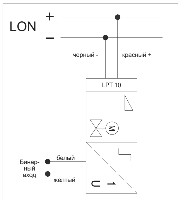
Схема подключения
